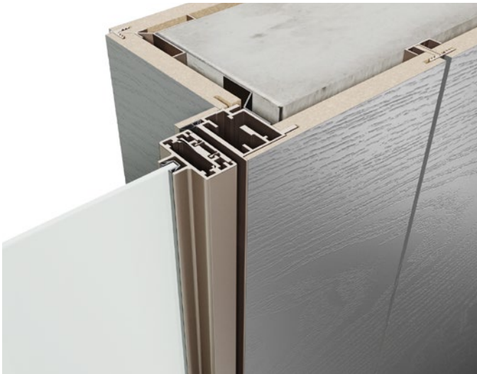
Otwieranie STANDARD OUT Opening
