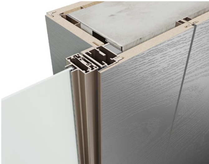
Otwieranie do wewnątrz IN Opening
